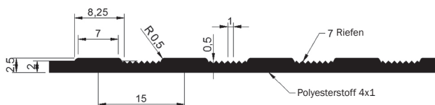
Rechteck/Riefen (MR)
